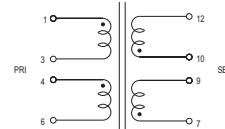
2. SCHEMATIC :
